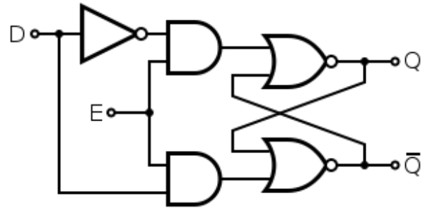
circuit de type bascule, permet de stocker 1 bit
